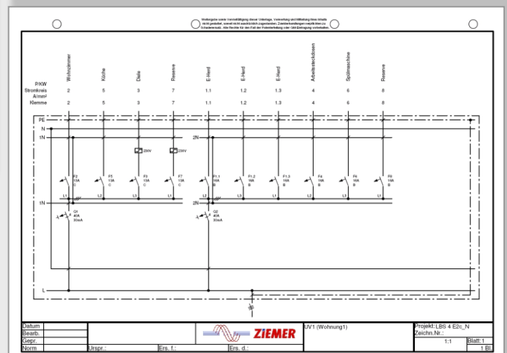
Übersichtsschaltplan im SCC-CAD Startup
